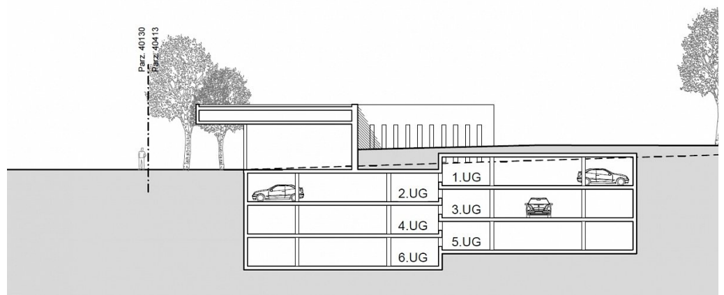
Querschnitt Tiefgarage
